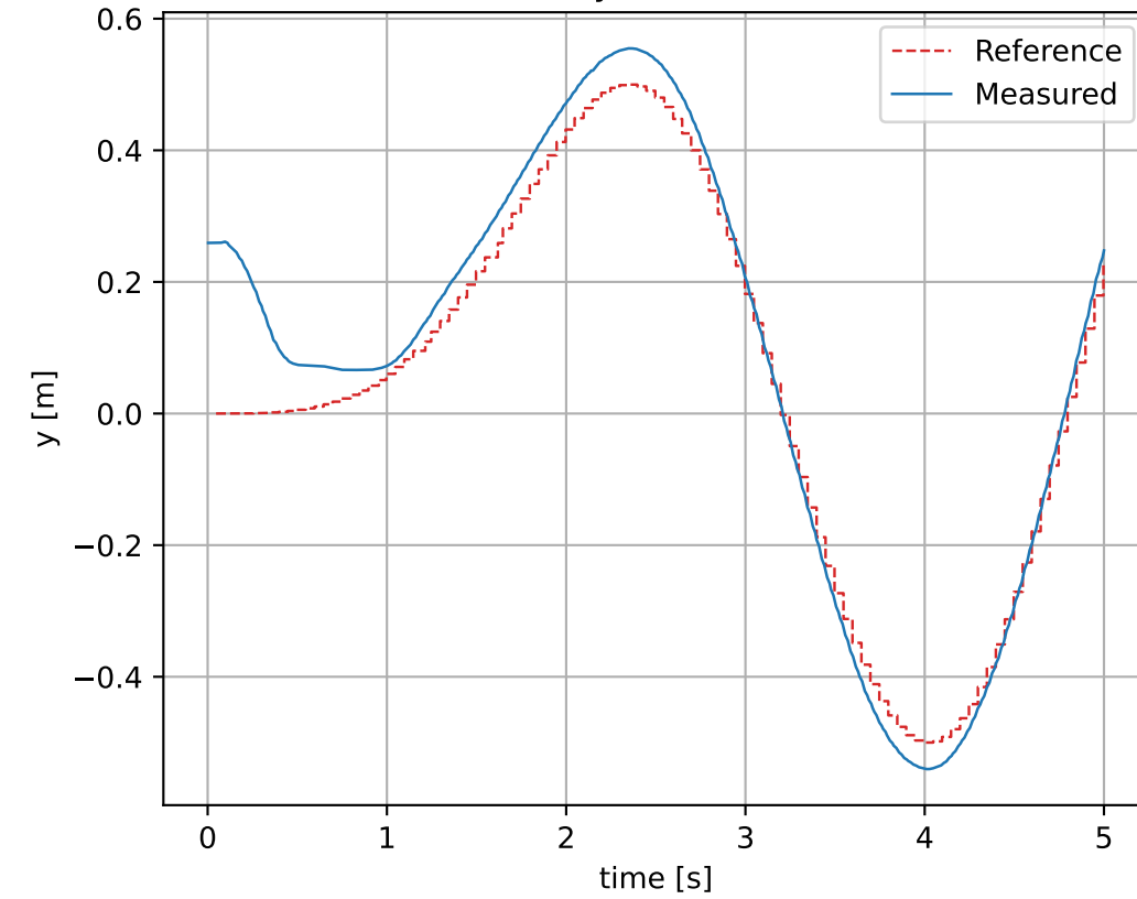
y State
